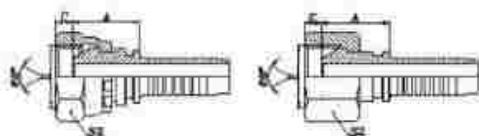
公制外内螺纹 60° METRIC FEMALE 60°CONE
